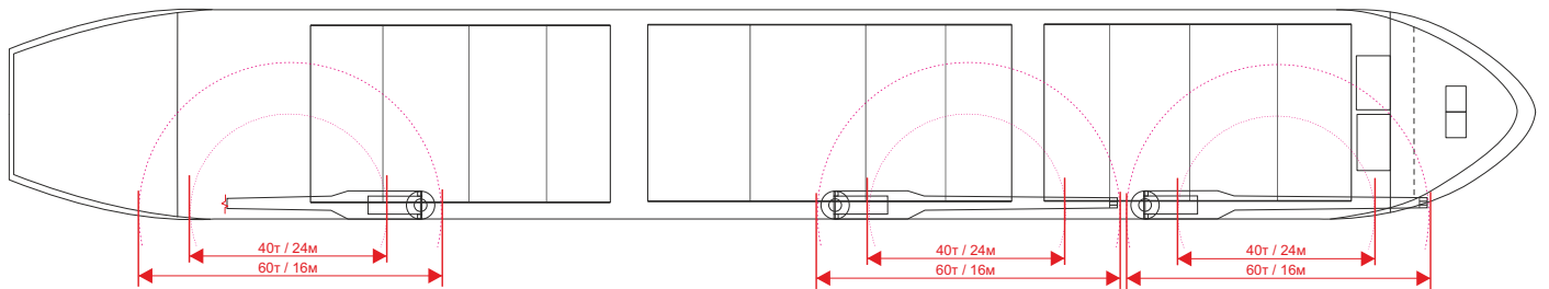
ГЛАВНАЯ ПАЛУБА
