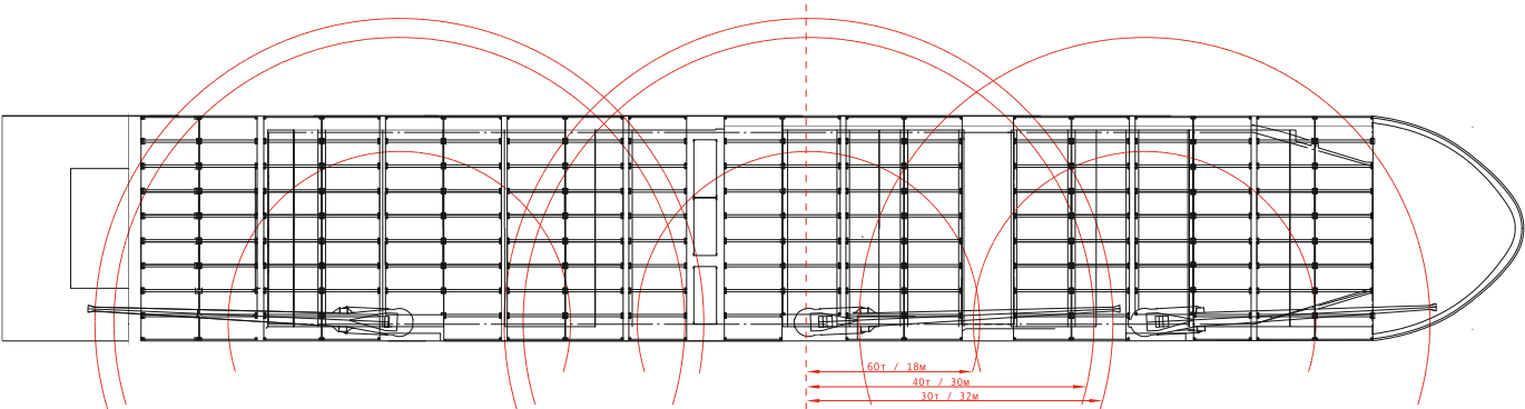
ГЛАВНАЯ ПАЛУБА/ КРЫШКИ ТРЮМА
