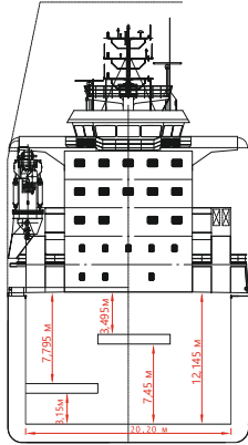
В РАЗРЕЗЕ
